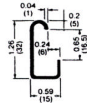
G rail EN 50035 - G 32
