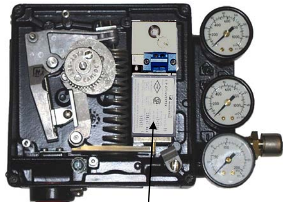
Siemens (Moore) 760E Positioner
