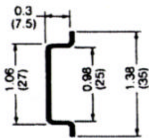
Cap rail EN 50022 - 35 x 7.5
