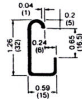
G rail EN 50035 - G 32
