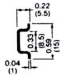
Cap rail EN 50045 - 15 x 5
